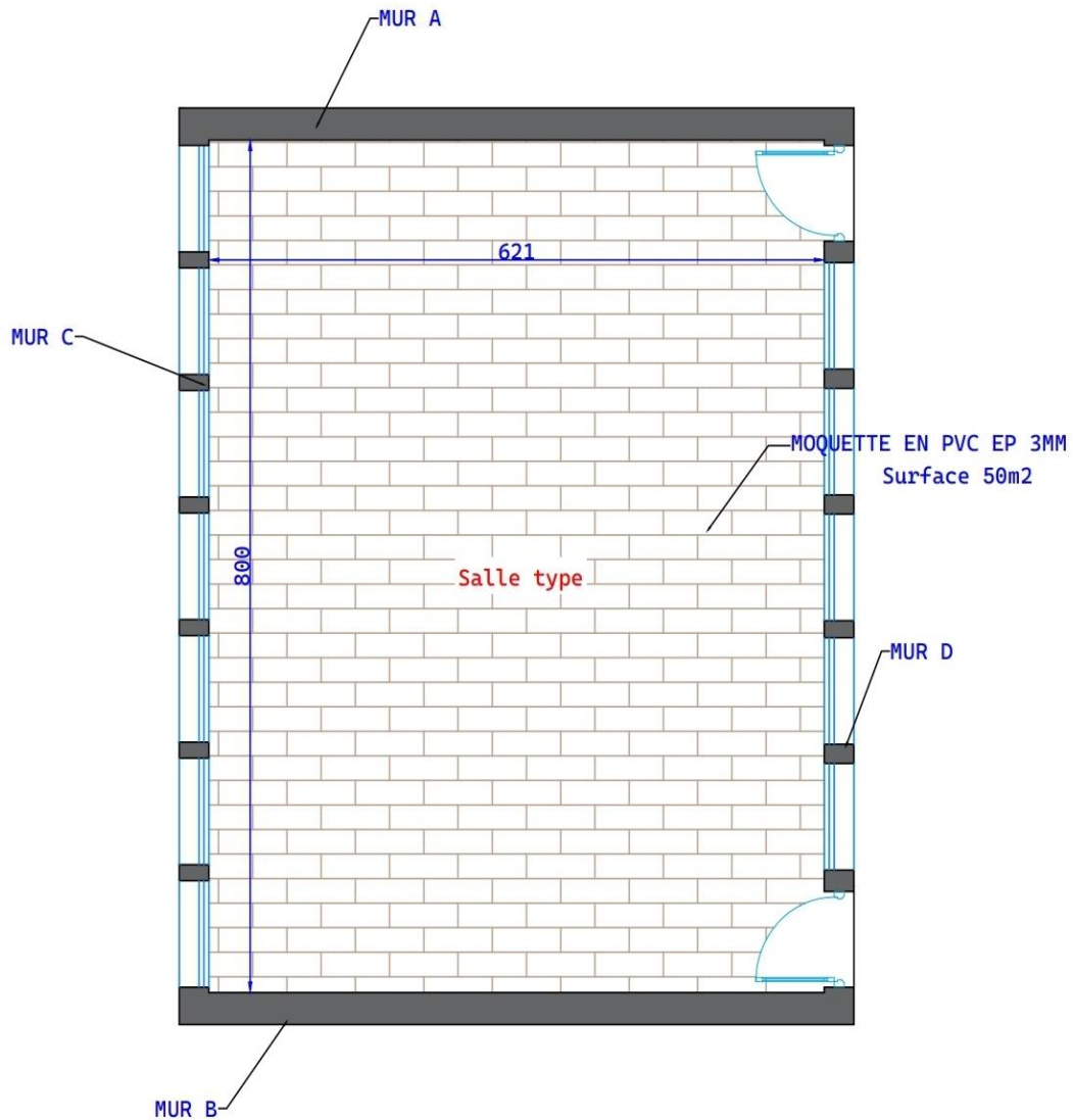
PLAN SALLE TYPE
