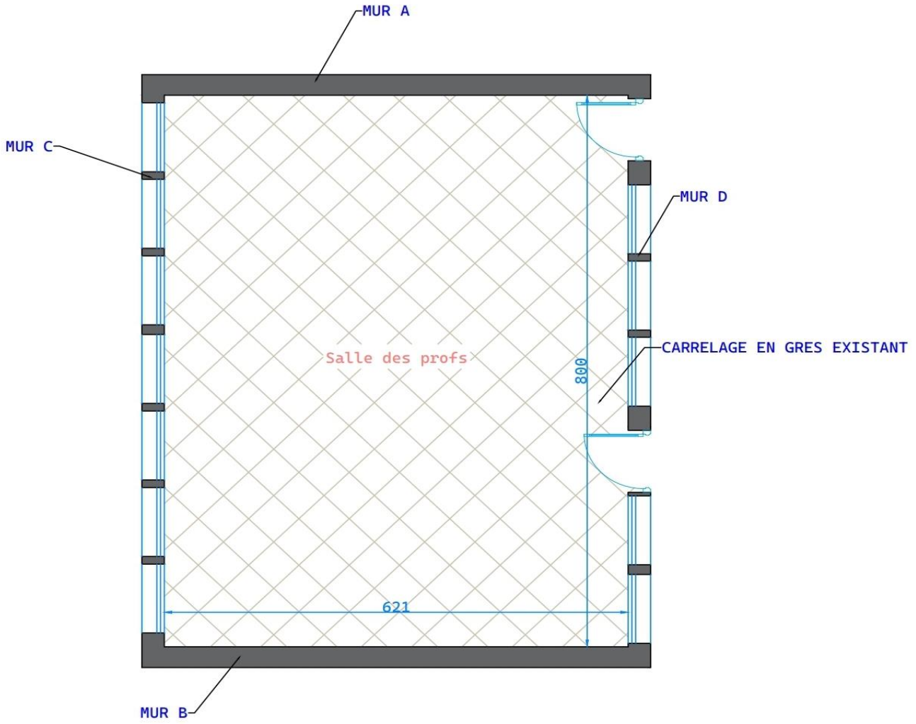
PLAN SALLE DES PROFS
